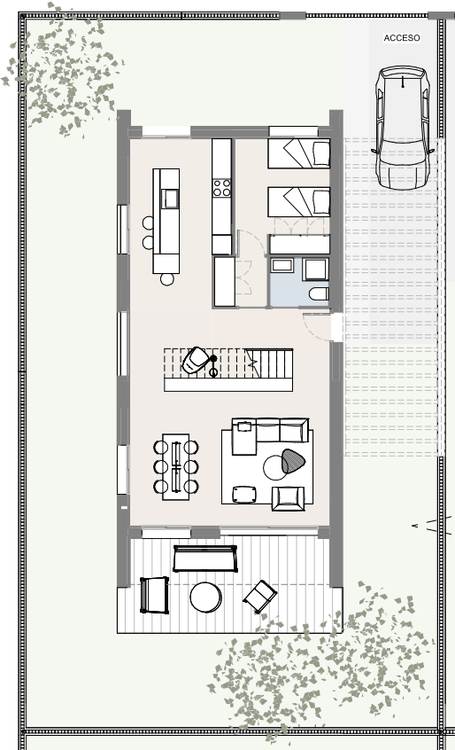
PLANTA BAJA
