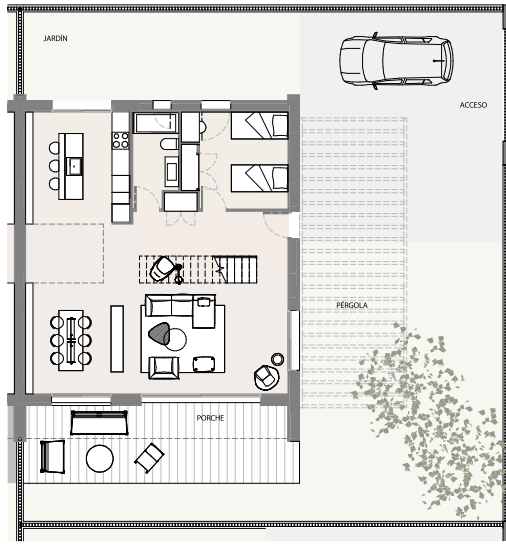
PLANTA BAJA
