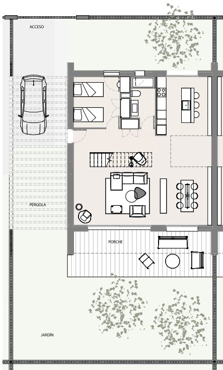
PLANTA BAJA
