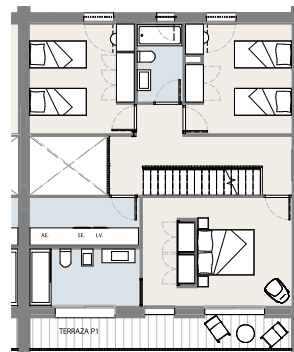
PLANTA PRIMERA
