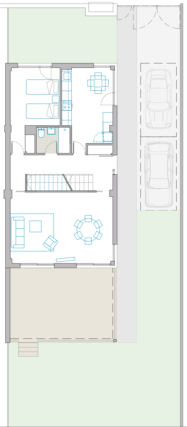
PLANTA BAJA
