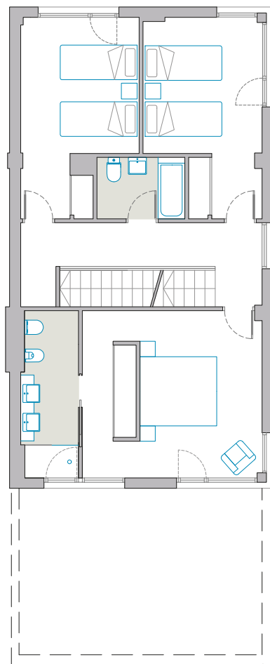
PLANTA PRIMERA
